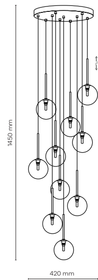
5944 / NILOS 10 x G9 / 230V / max 6W / LED KL / 7525 (ø 120mm)
