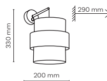
5956 / CALISTO 1 x E27 / 230V / max 15W / LED AB 9507 / 9506 5956 5955
